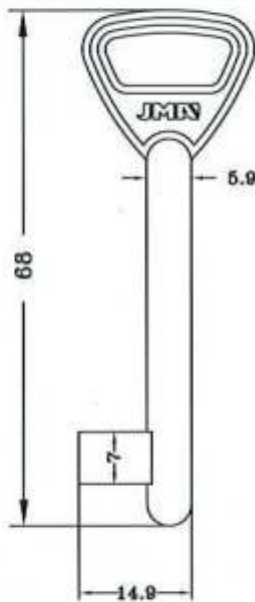
CHU-4G LAITON
