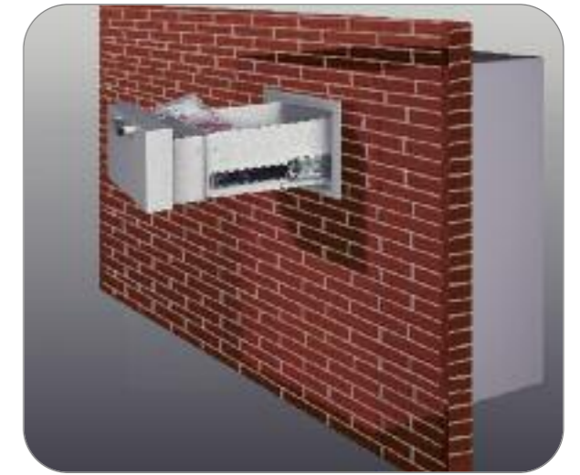
Modèle Zephir Dépôt 1002. Avec tiroir déporté vers l'arrière pour traverser un mur de 100 mm.
